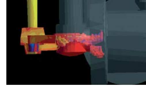
Valf döküm dolulumunun simülasyonu
