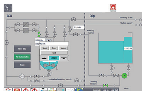
Automatizovaná Inteligentní nátěrová jednotka firmy Foseco: Sleduje hustotu nátěru v reálném čase, a proto nabízí lepší konzistenci z hlediska tloušťky mokré vrstvy.
